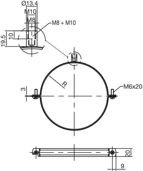
Ø80 - Ø400
